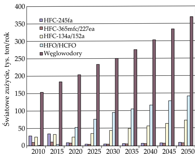
Rys. 3. Prognoza potencjalnego wzrostu światowego zapotrzebowania (t/r.) na HFC i zamienniki (substancje HFO i HCFO oraz węglowodory) w piankach (w tym piankach PUR i ekspandowanym polistyrenie XPS) do 2050 r., przy założeniu niewycyfywania HFC, w podziale na rodzaje czynników spienających (na podstawie [17])
